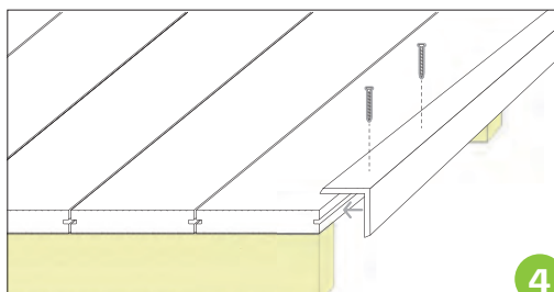
Montering av gop Woodlon Kantprofil.
